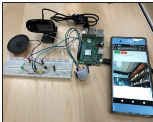
圖 2：多功能智慧燈之示意圖
